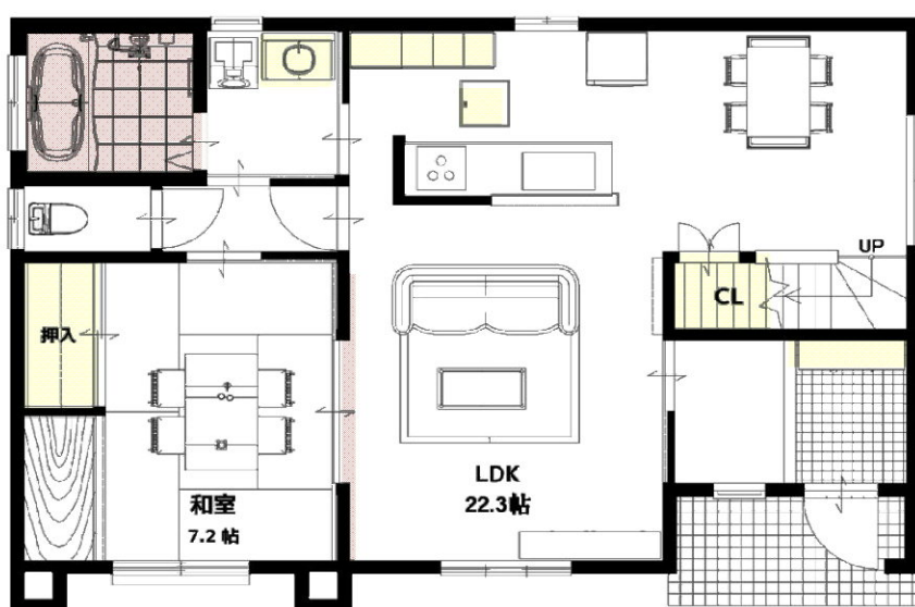
1F 平面図
