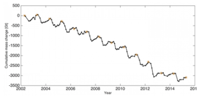
グリーンランドの水床量の推移
