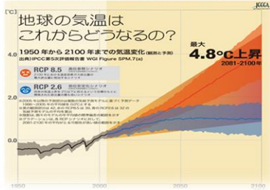
2100年の気温変化の予測
